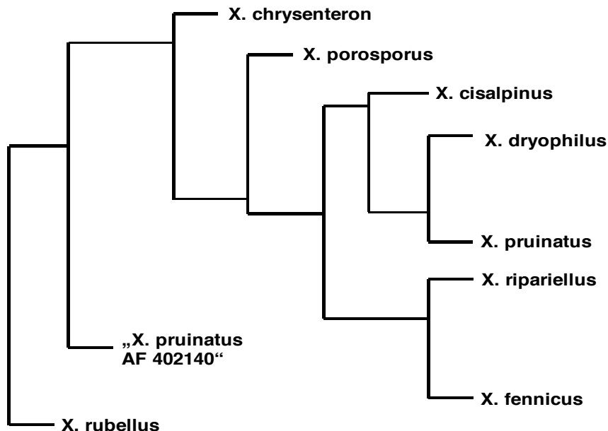
Abb. 2: Xerocomellus ("Chrysenteron-Gruppe"); vereinfachte Darstellung nach Peintner et al., 2003
