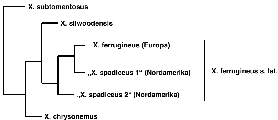
Abb. 1: Xerocomus s. str.; vereinfachte Darstellung nach Taylor et al. 2006, 2007
